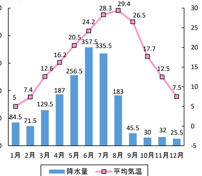
(mm) 令和5年 平均気温及び降水量 (℃)
