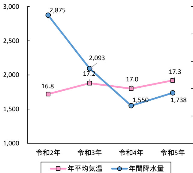
(mm) 年平均気温及び年間総降水量の推移 (℃)
